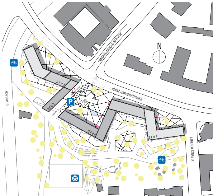
LAGEPLAN
